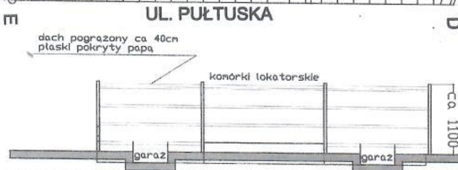
SCHEMAT PRZEKROJU POPRZECZNEGO
